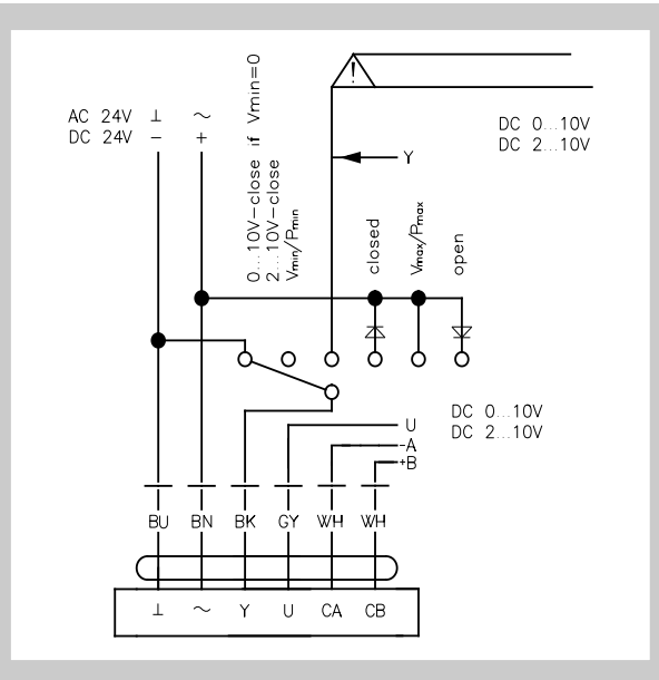
Fig. 24 Regulators GUAC-...-MB
