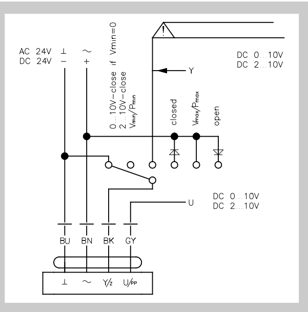
Fig. 23 Regulators GUAC-...
